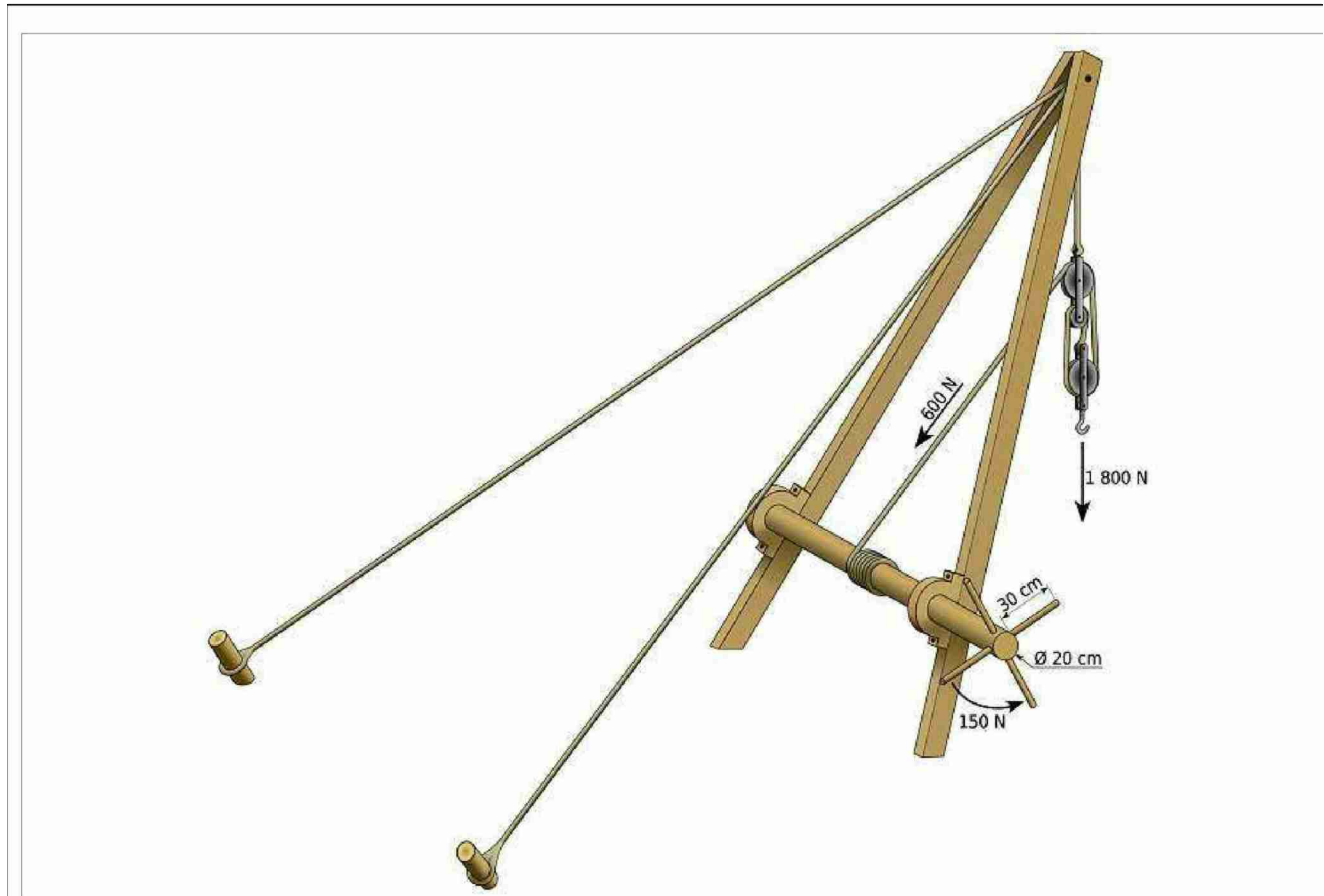
Ausgeklügelt. Den griechischen Kran Trispastos (3-Rollen-Zug) könnte man auch heute noch bauen.
